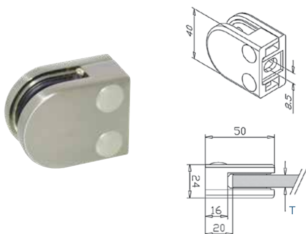
Pinces à verre modèle 00 - Plat S
