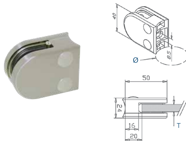
Pinces à verre modèle 00 - Tube S
